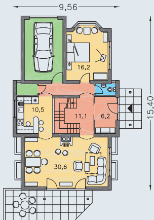
PRÍZEMIE [plocha 101.3 m 2 ]
