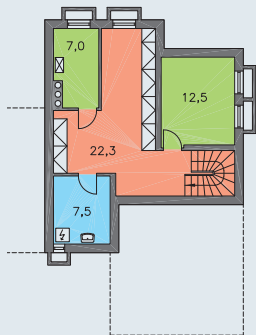
SUTERÉN [plocha 55.8 m 2 ]
