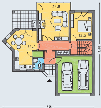
PRÍZEMIE [plocha 104.9 m 2 ]
