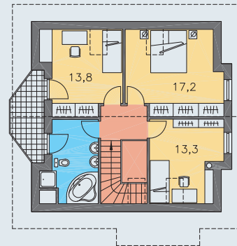
POSCHODIE [plocha 62.5 m 2 ]
