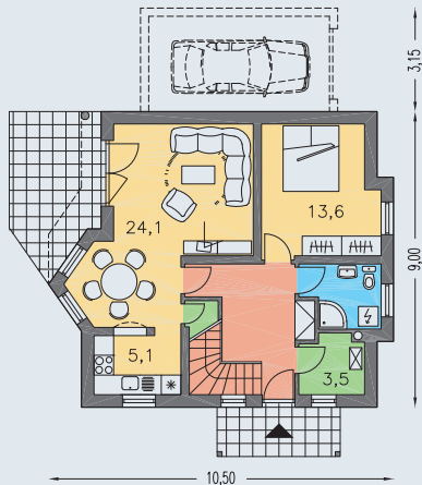
PRÍZEMIE [plocha 65.5 m 2 ]
