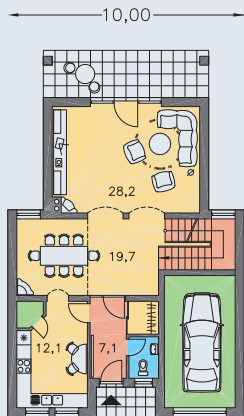
PRÍZEMIE [plocha 93.8 m 2 ]
