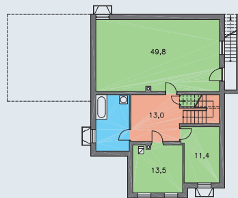
SUTERÉN [plocha 1006.5 m 2 ]
