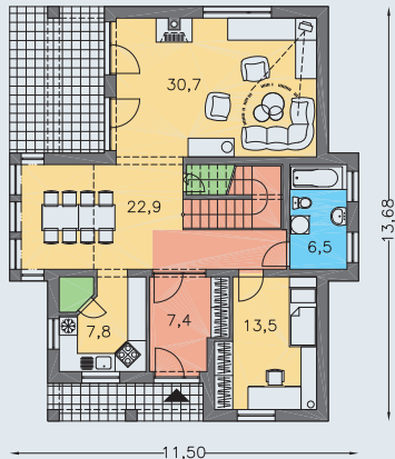
PRÍZEMIE [plocha 100.1 m 2 ]
