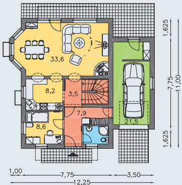
PRÍZEMIE [plocha 91.7 m 2 ]
