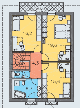
POSCHODIE [plocha 71.8 m 2 ]
