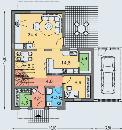
PRÍZEMIE [plocha 82.2 m 2 ]
