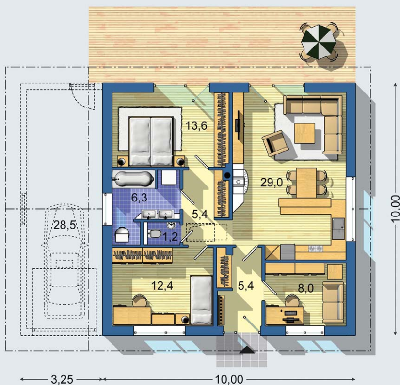
PRÍZEMIE [celková plocha 81.3 m 2 ]
