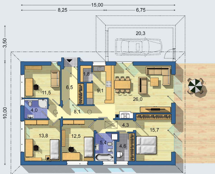
PRÍZEMIE [celková plocha 123.3 m 2 ]
