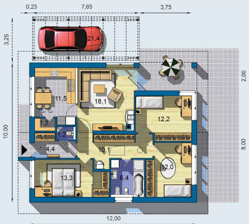
PRÍZEMIE [celková plocha 90.6 m 2 ]
