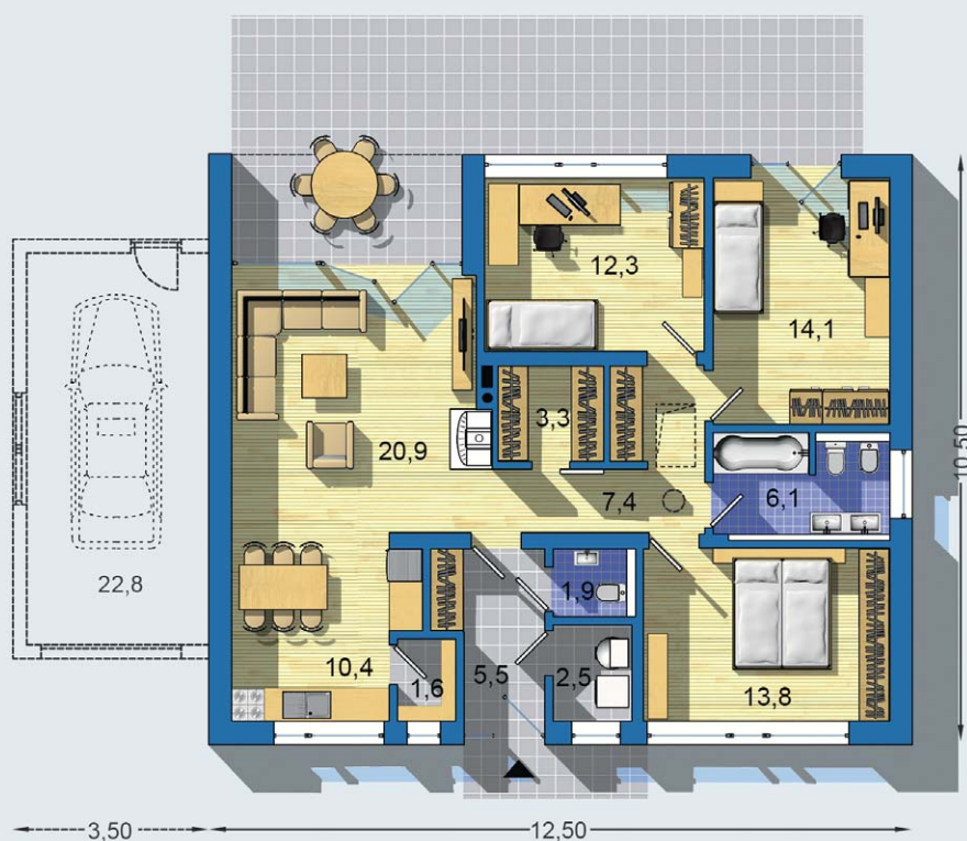
PRÍZEMIE [celková plocha 99.8 m 2 ]
