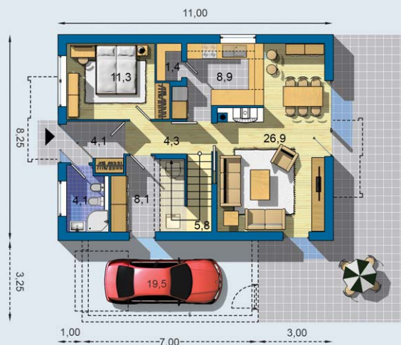
PRÍZEMIE [celková plocha 74.7 m 2 ]
