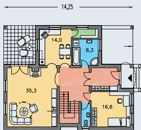
PRÍZEMIE [plocha 104.1 m 2 ]
