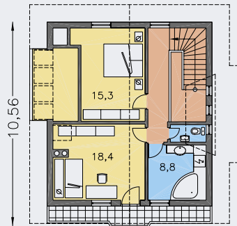
POSCHODIE [plocha 58.7 m 2 ]
