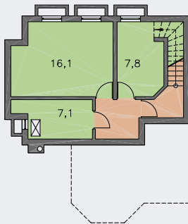
SUTERÉN [plocha 42.8 m 2 ]
