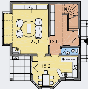
PRÍZEMIE [plocha 62.2 m 2 ]
