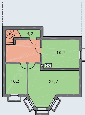
SUTERÉN [plocha 71.3 m 2 ]
