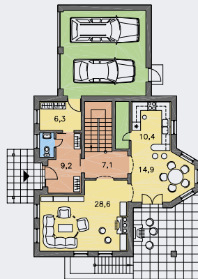
PRÍZEMIE [plocha 122.0 m 2 ]
