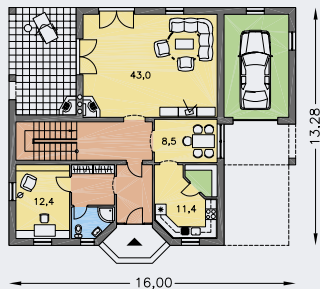
PRÍZEMIE [plocha 130.3 m 2 ]
