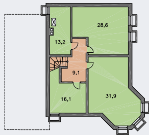
SUTERÉN [plocha 102.7 m 2 ]
