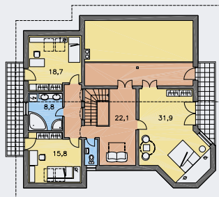
POSCHODIE [plocha 140.8 m 2 ]
