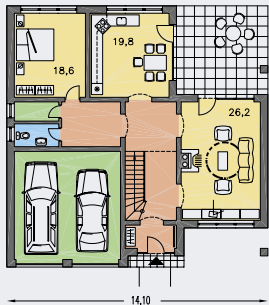
PRÍZEMIE [plocha 133.3 m 2 ]
