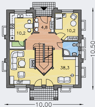
PRÍZEMIE [plocha 76.1 m 2 ]
