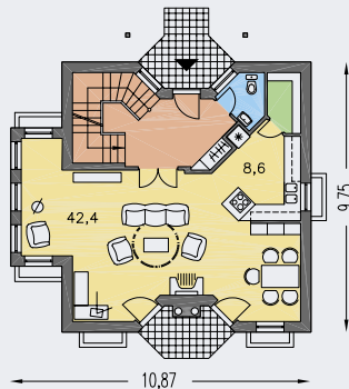
PRÍZEMIE [plocha 70.6 m 2 ]
