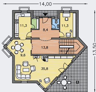
PRÍZEMIE [plocha 103.8 m 2 ]
