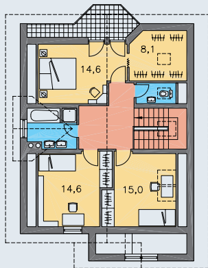
POSCHODIE [plocha 77.3 m 2 ]
