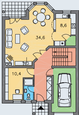
PRÍZEMIE [plocha 92.4 m 2 ]
