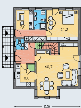
PRÍZEMIE [plocha 100.5 m 2 ]
