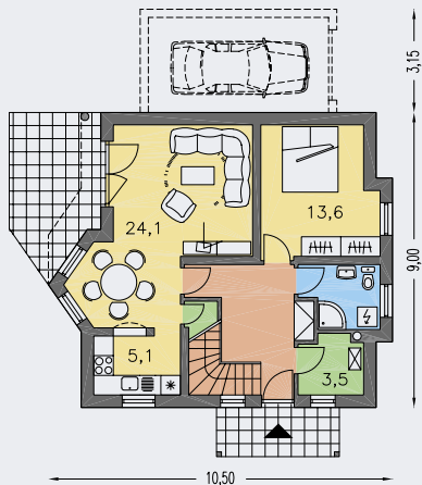
PRÍZEMIE [plocha 65.5 m 2 ]
