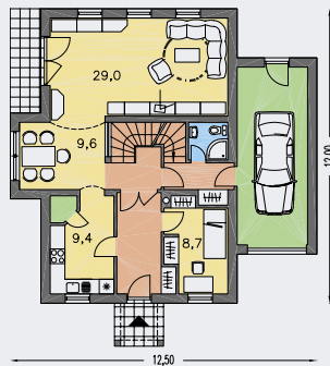
PRÍZEMIE [plocha 99.2 m 2 ]
