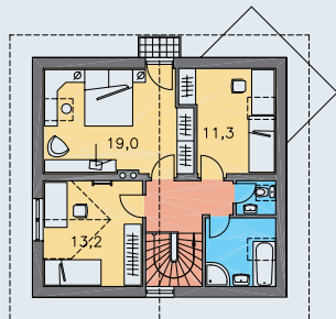
POSCHODIE [plocha 57.3 m 2 ]
