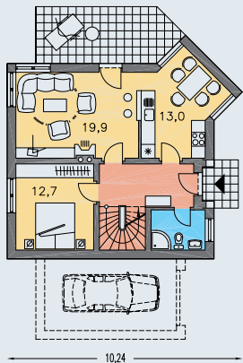
PRÍZEMIE [plocha 61.1 m 2 ]
