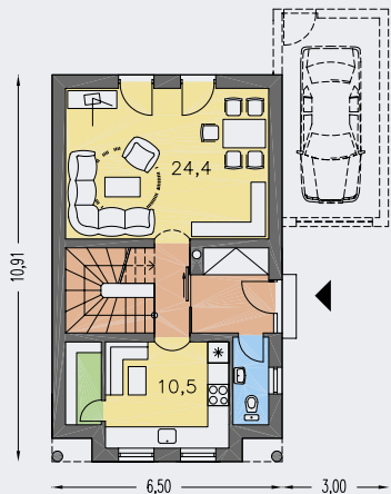
PRÍZEMIE [plocha 53.2 m 2 ]
