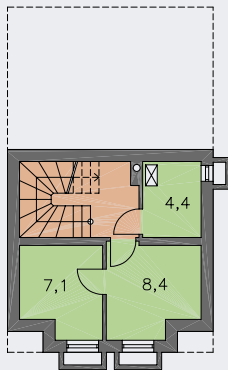
SUTERÉN [plocha 31.9 m 2 ]
