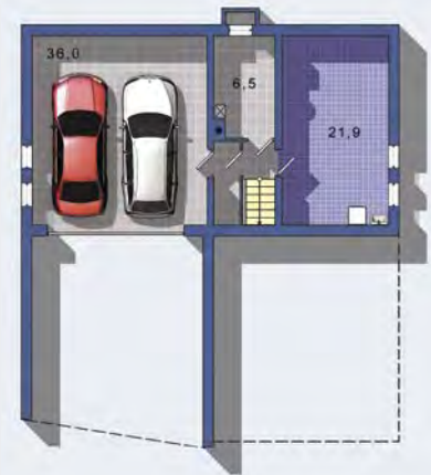
SUTERÉN [celková plocha 71.0 m 2 ]
