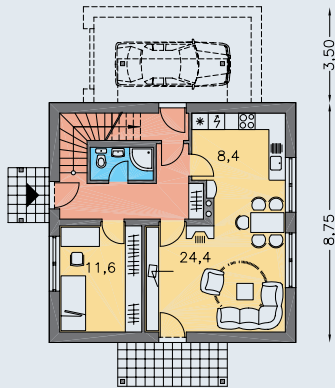
PRÍZEMIE [plocha 62.1 m 2 ]
