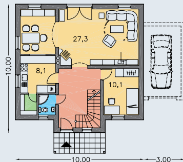
PRÍZEMIE [plocha 75.2 m 2 ]
