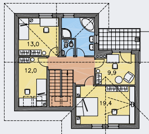
POSCHODIE [plocha 80.5 m 2 ]
