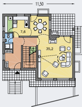
PRÍZEMIE [plocha 79.4 m 2 ]
