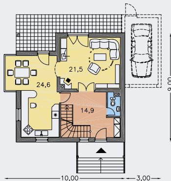
PRÍZEMIE [plocha 73.2 m 2 ]
