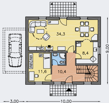
PRÍZEMIE [plocha 72.3 m 2 ]
