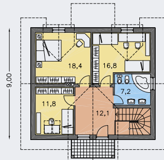
POSCHODIE [plocha 71.4 m 2 ]
