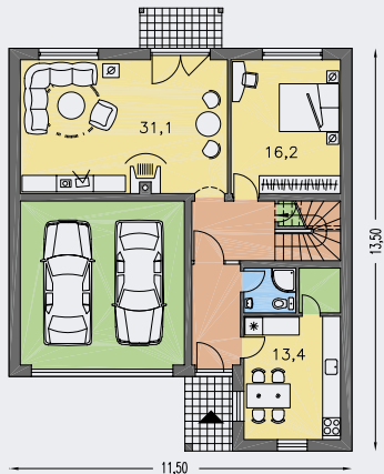
PRÍZEMIE [plocha 113.1 m 2 ]
