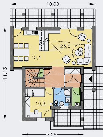
PRÍZEMIE [plocha 73.1 m 2 ]
