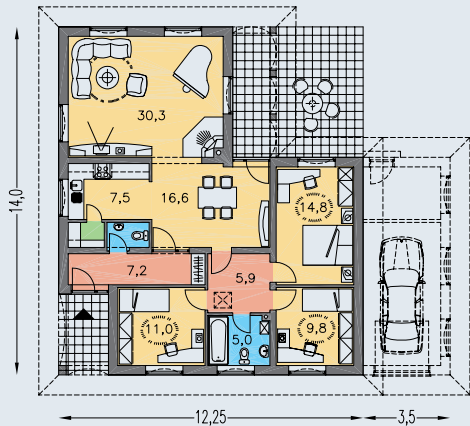
PRÍZEMIE [plocha 111.3 m 2 ]
