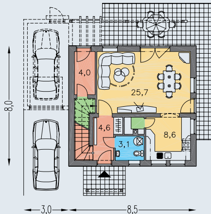
PRÍZEMIE [plocha 52.2 m 2 ]
