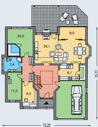
PRÍZEMIE [plocha 162.7 m 2 ]
