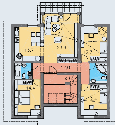
POSCHODIE [plocha 111.0 m 2 ]
