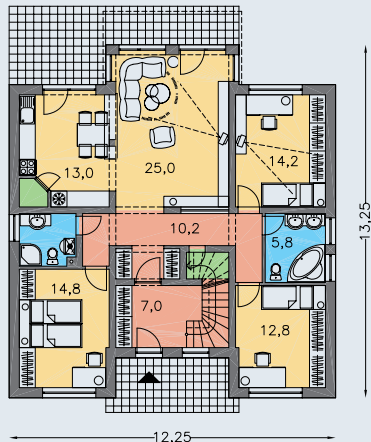
PRÍZEMIE [plocha 118.4 m 2 ]
