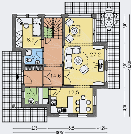
PRÍZEMIE [plocha 76.9 m 2 ]
