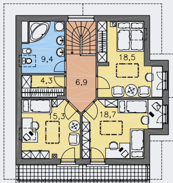
POSCHODIE [plocha 84.1 m 2 ]
