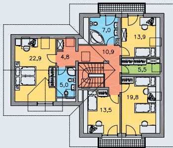
POSCHODIE [plocha 125.0 m 2 ]
