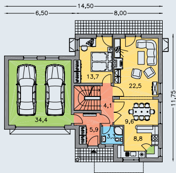
PRÍZEMIE [plocha 127.0 m 2 ]
