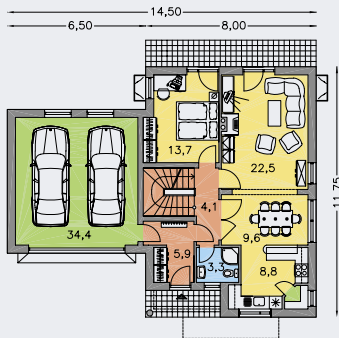
PRÍZEMIE [plocha 108.0 m 2 ]
