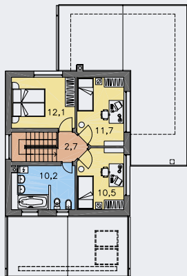
POSCHODIE [plocha 47.3 m 2 ]
