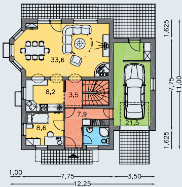
PRÍZEMIE [plocha 91.7 m 2 ]
