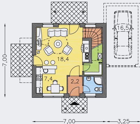
PRÍZEMIE [plocha 39.1 m 2 ]
