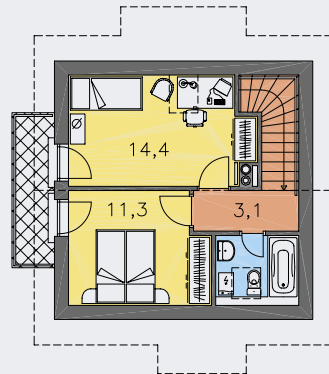
POSCHODIE [plocha 38.0 m 2 ]
