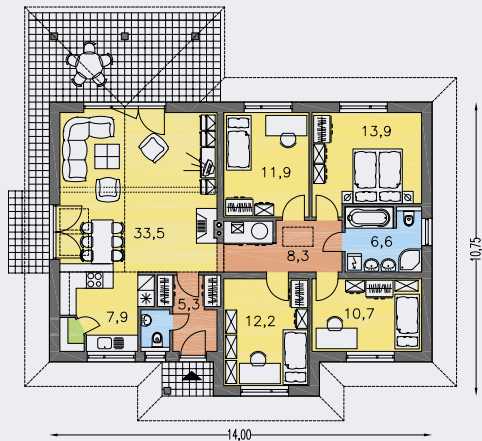
PRÍZEMIE [plocha 112.7 m 2 ]
