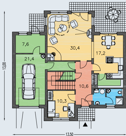
PRÍZEMIE [plocha 121.0 m 2 ]
