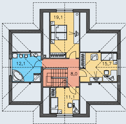
POSCHODIE [plocha 66.0 m 2 ]
