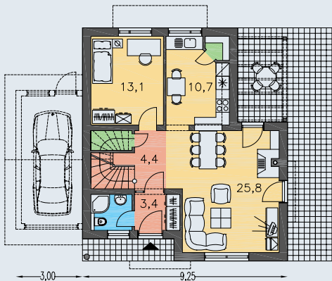
PRÍZEMIE [plocha 67.7 m 2 ]
